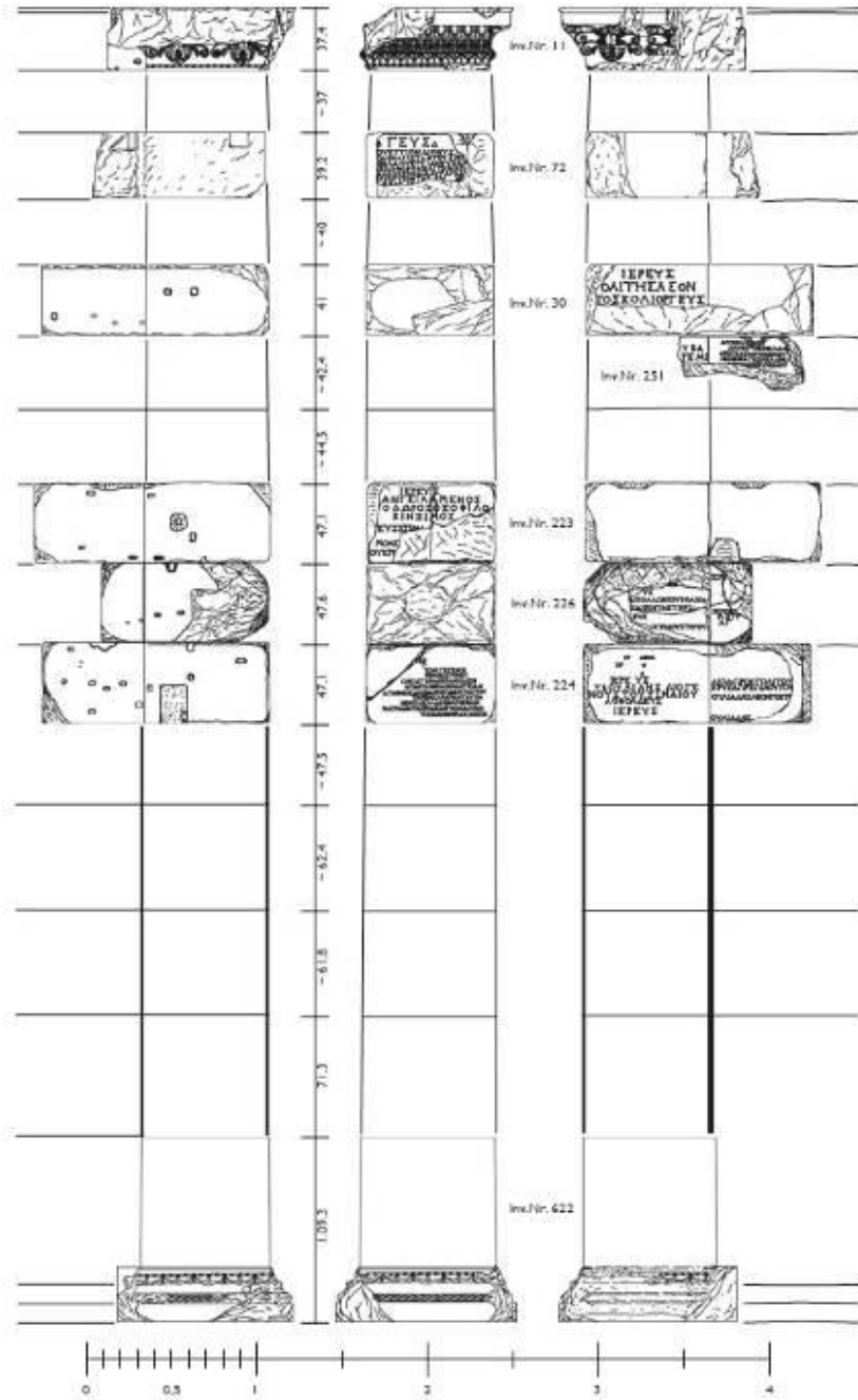
Çizim 4- Lagina Hekate Tapınağı Sağ Anta (Brize vd. 2023, Abb. 2)
