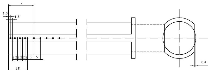
Sertleştirilmiş deney numunesinin sertliğini ölçmek için, uzunluk eksenini doğrultusunda birbirinden 180° açıklıkta karşılıklı iki yüzey taşlanır. Taşlama derinliği 0,4 mm olmalıdır, Şekil 1.3 . Taşlama yapılması sırasında deney numunesinin aşırı ısınarak mikro yapısının değişmemesi için, bol miktarda soğutucu verilmelidir. Taşlama sırasında yumuşama olmamasına dikkat edilmelidir. Bunun için deney numunesi % 5’lik nitrik asit çözeltisi içinde kararınca kadar tutulur. Sıcak suda yıkandıktan sonra 2 veya 3 saniye % 50’lik seyreltik hidroklorik asit çözeltisine batırılır. Sıcak suda tekrar yıkanarak sıcak hava ile kurutulur. Deney parçası uygun bir taşıyıcıya yerleştirilerek, hazırlanmış yüzeylerin uzunluk eksenleri boyunca Rockwell C sertlik ölçümleri yapılmalıdır. Rockwell C sertlik ölçümü yerine 30 kgf yükü Vickers sertlik ölçümü de yapılabilir. İkinci taşlanmış yüzeyde sertlik deneyi yapılmadan önce birinci yüzeydeki batıcı uç iz çıkıntılarının taşlanması yapılmalıdır. Ölçme noktalarının yerleri Şekil 3 ’e uygun olacak şekilde yapılmalıdır. Sertlik ölçümleri su vermenin yapıldığı alından başlanarak 1,5-1,5-2-2-2-2-2 mm olan mesafelerde yapılır. Toplam 15 mm’yi bulan bu noktalardan sonra 5’er mm aralıkla ölçümler yapılır. Elde edilen farklı mesafelerdeki sertlik değerleri bir grafiğe taşınırsa malzemenin Jominy sertleştirilebilirlik eğrisi elde edilmiş olur.
