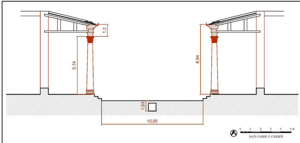
Çizim 2: Batı Cadde, portikler ve kanalizasyonun restitüsyon kesiti
