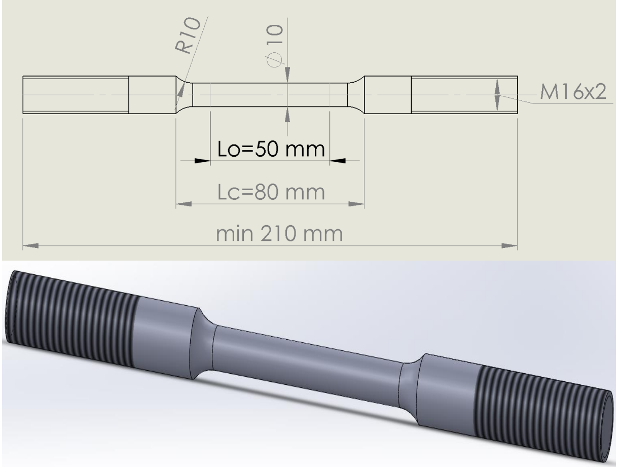
Şekil 1.6. 10 mm numune çapı için numune boyutları ve katı modeli
