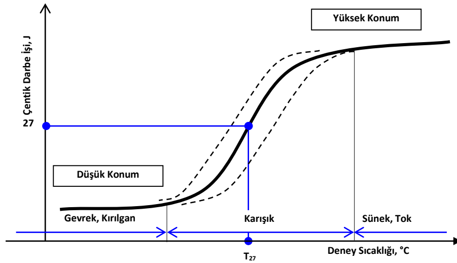
Şekil 2.5: Geçiş sıcaklığı ( T_{27} ) olan bir malzemenin çentik darbe işi – deney sıcaklığı diyagramı
