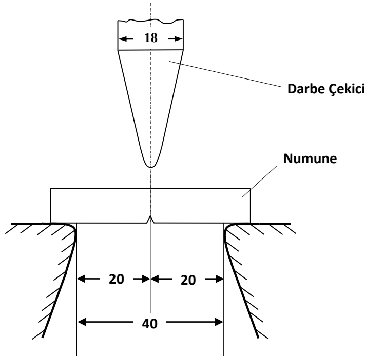
Şekil 2.3: Charpy çentik darbe deneyinde çekik ve numunenin makine üzerindeki yerleşimi
