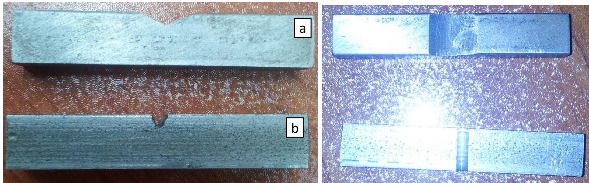
Şekil 2.6: Gereğinden fazla geniş açıda (a) ve gereğinden derin ve şekilsiz (b) açılmış çentiklere ait görünüm
