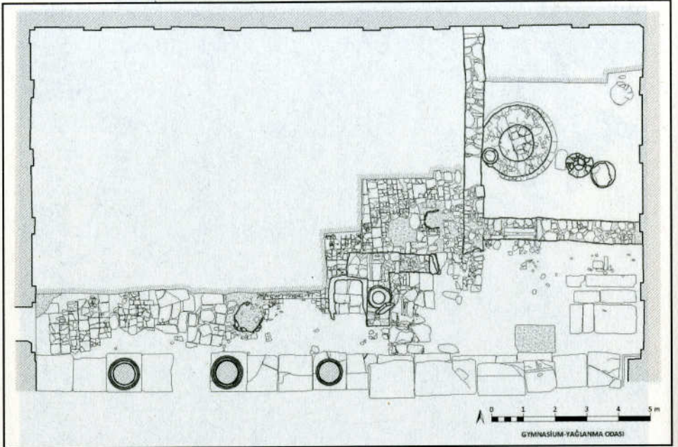
Çizim 2: Gymnasium yağlanma odası ve bulunan kalıntıların rölöve çizimi
