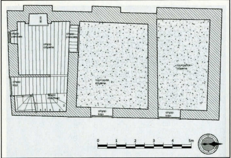
Çizim 5: Hüseyin Gürkan Evi (1247 parsel) zemin kat restitüsyon planı
