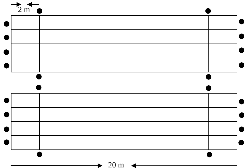
Şekil 1: Dayanıklılık Testi Parkuru
