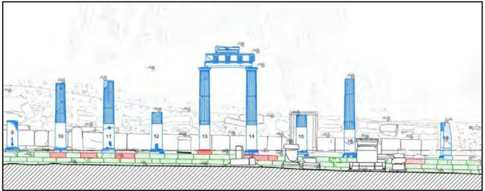
Çizim 1: Lagina Kuzey Stoa restorasyon projesinden cephe görünüşü.
